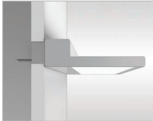
DRYWALL FLANGE 0.625"
